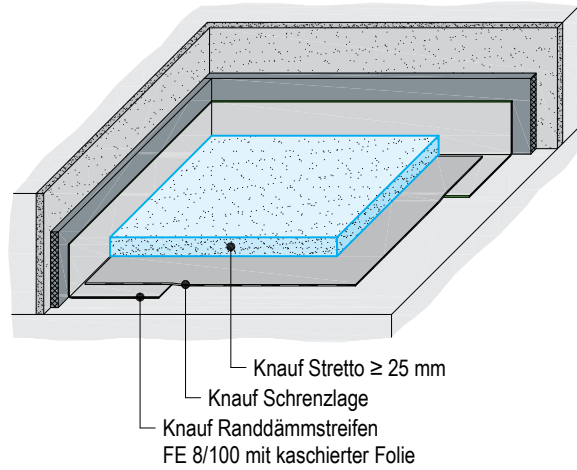
Knauf Stretto auf Trennschicht
