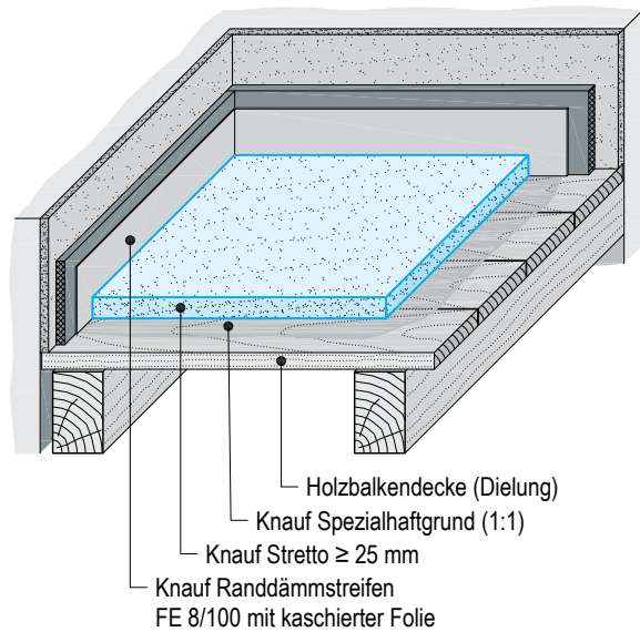
Knauf Stretto auf Dielung
